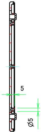
E-E ( 1 : 3 )
